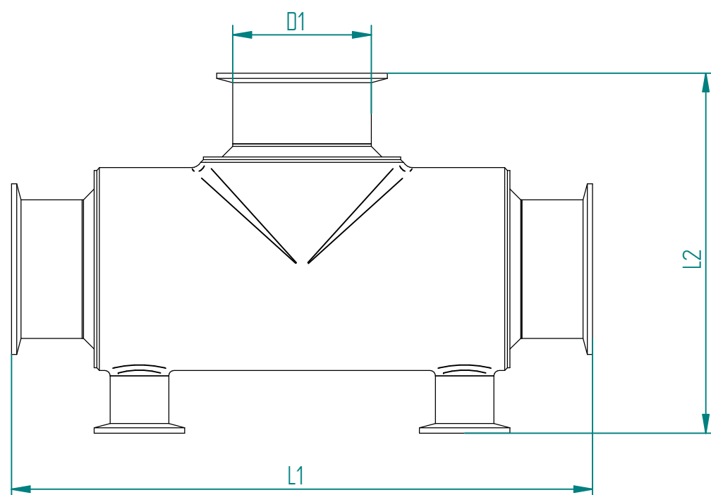
VISTA LATERALE
