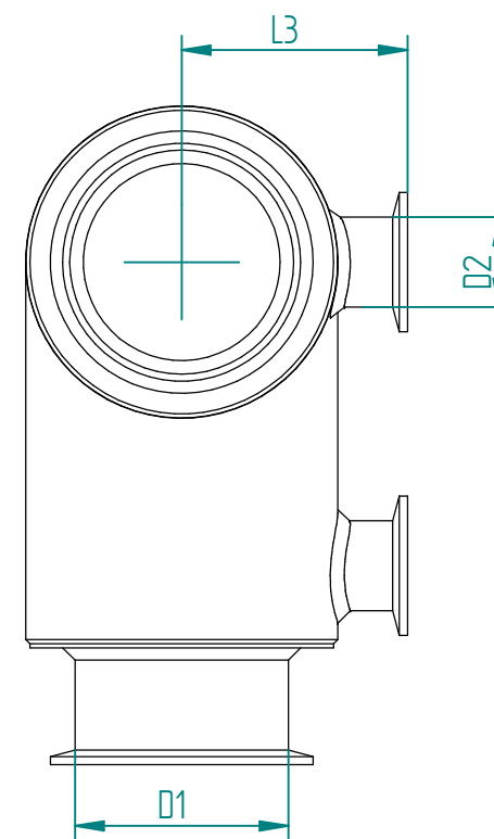
VISTA FRONTALE
